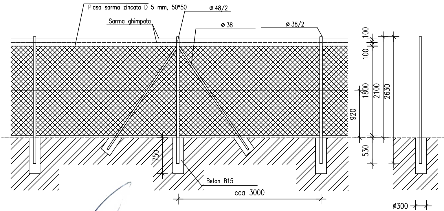
Detalii imprejmuire
