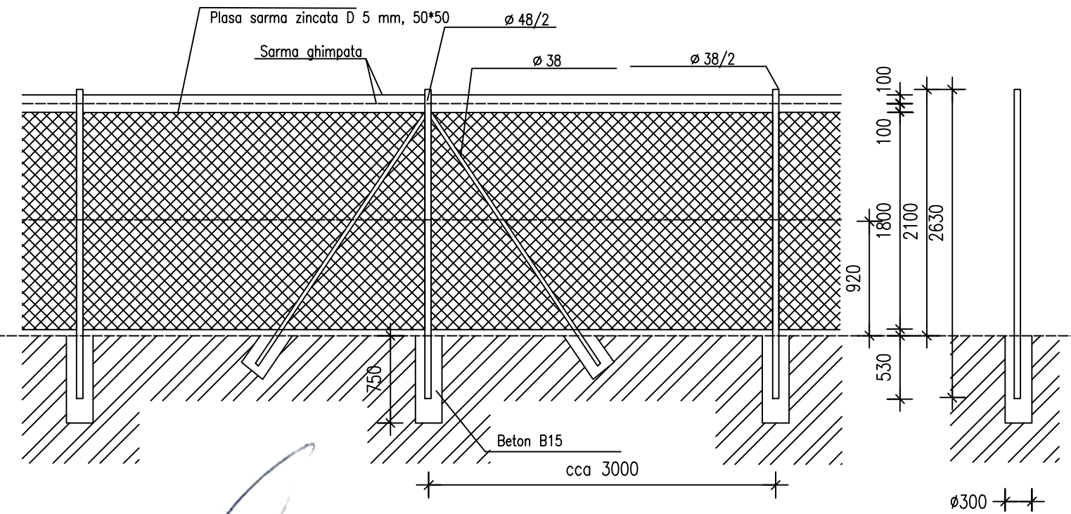
Detalii imprejmuire
